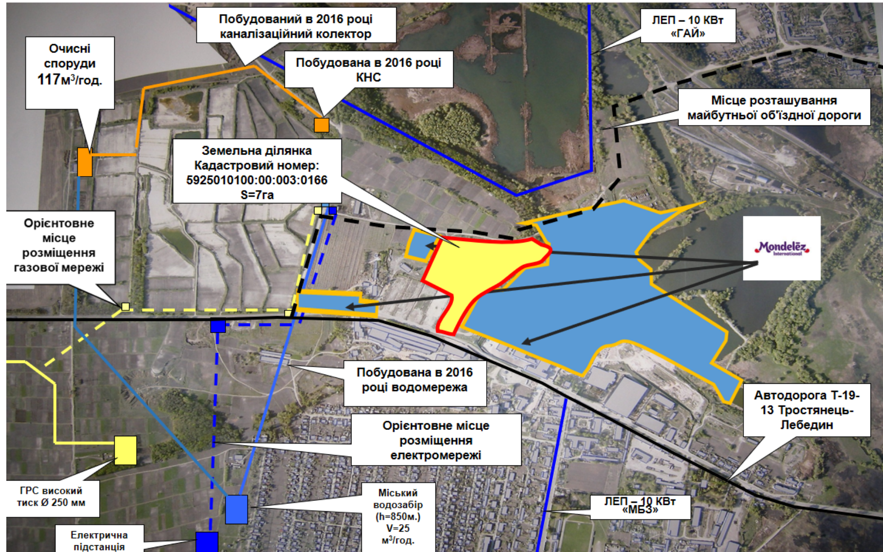
Схема розміщення земельної ділянки кадастровий номер 5925010100:00:003:0166 з існуючими комунікаціями
